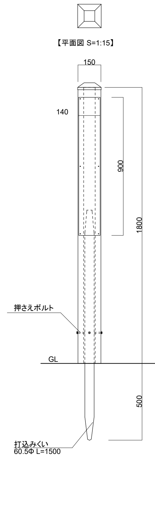
【打込みくいタイプ】
