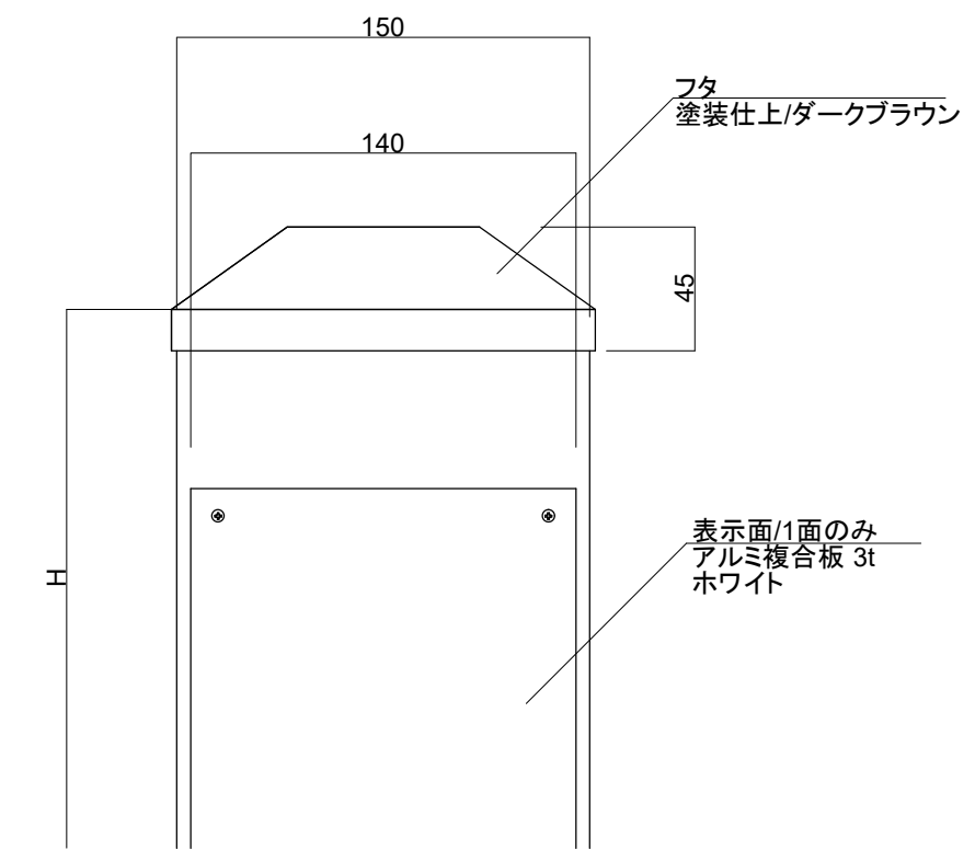
【正面図 S=1:3】
