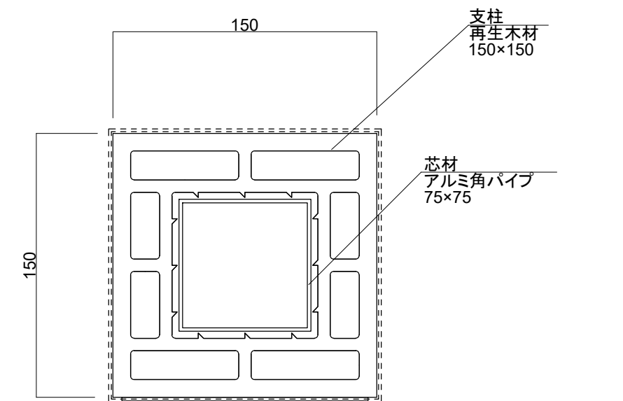
【断面図 S=1:3】
