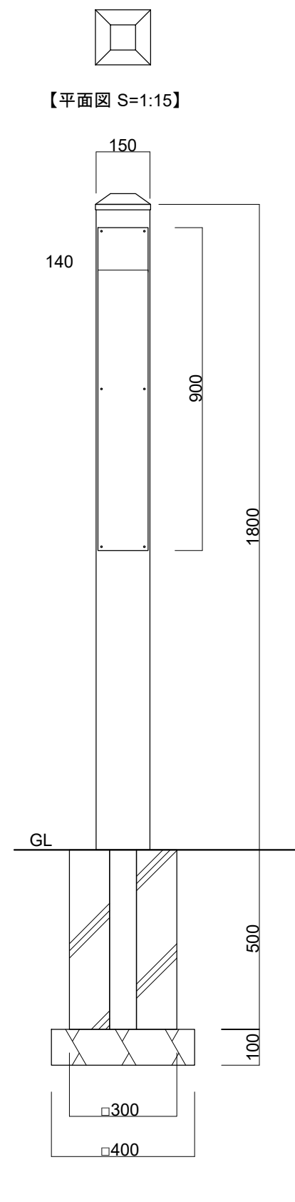
【基礎タイプ】
