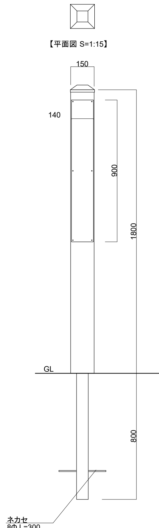
【土中タイプ】
