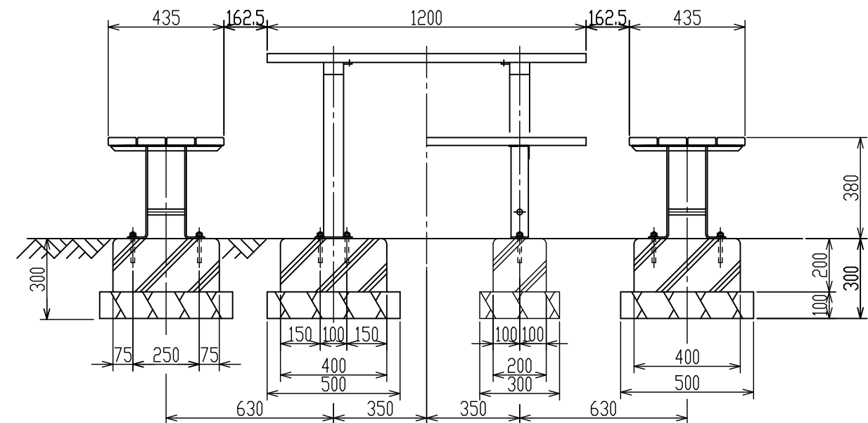
B-B矢視図
