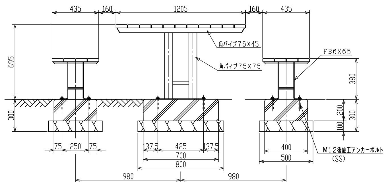
A-A矢視図
