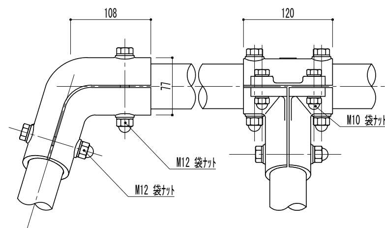
梁部詳細図 S=1/5
