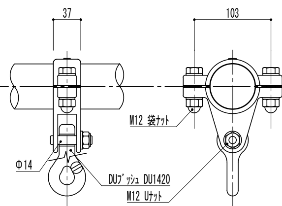
ハンガー取付け詳細図 S=1/5
