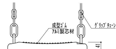
座板取付部詳細図 S=1/10
