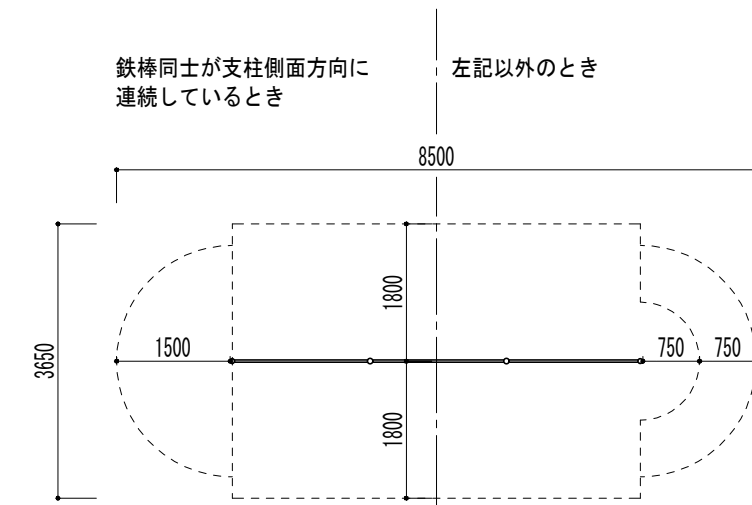
安全領域図 S=1/100
