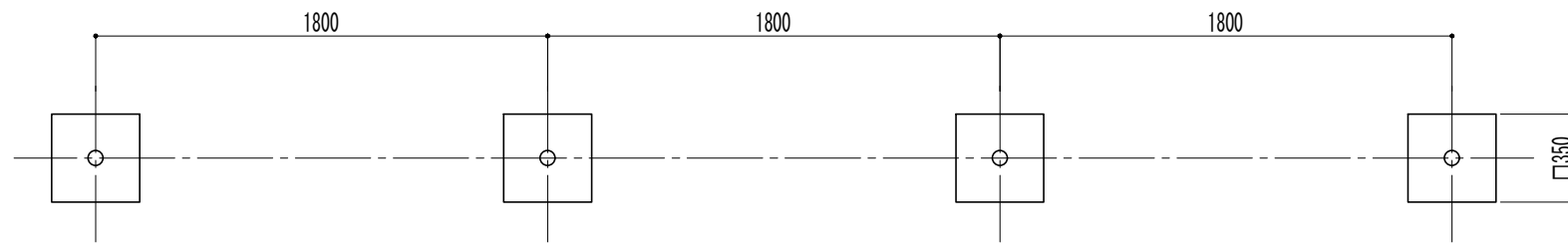
基礎伏図
