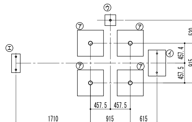
基礎伏図
