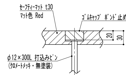
セーフティマット詳細図
