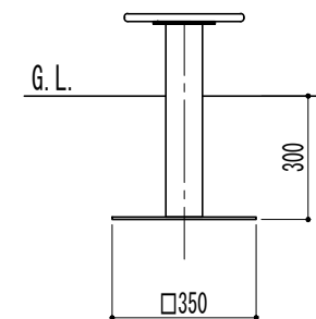
ステップ詳細図
