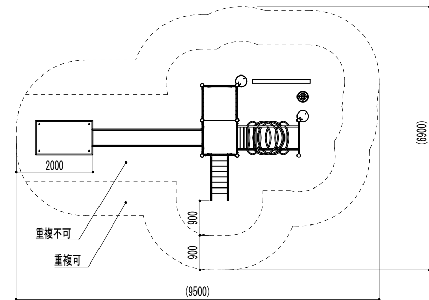
安全領域図 S=1/100
