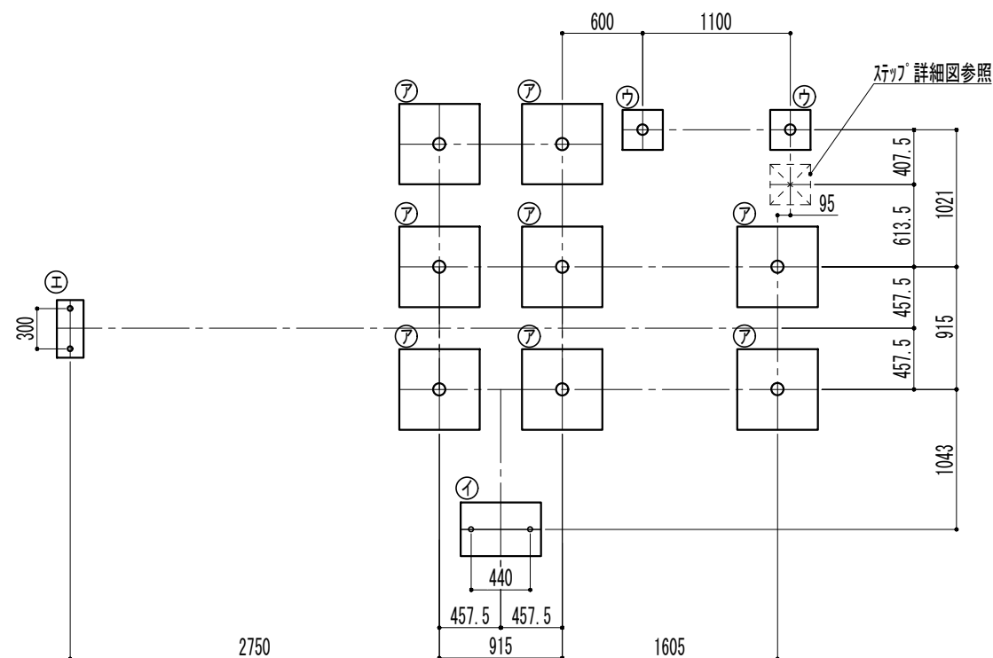
基礎伏図
