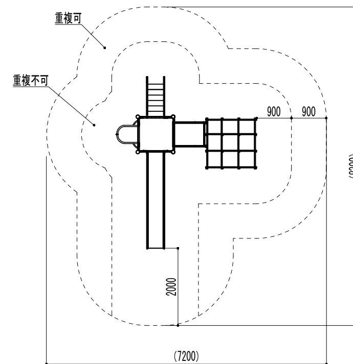
安全領域図 S=1/100
