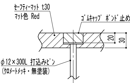
セーフティーマット詳細図
