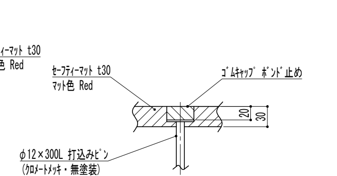
セーフティマット詳細図
