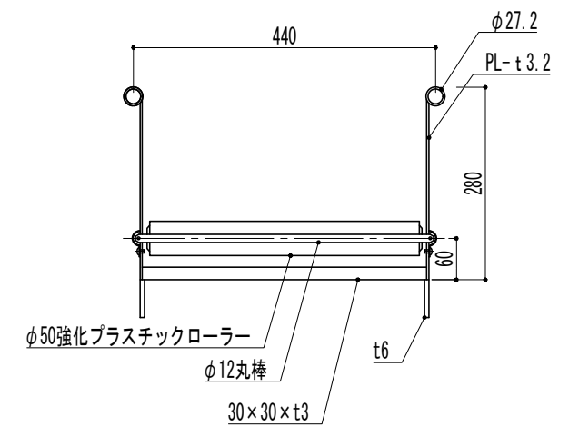
滑面断面図 S=1/10
