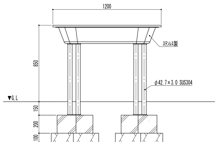
正面図
