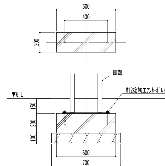
基礎詳細図
