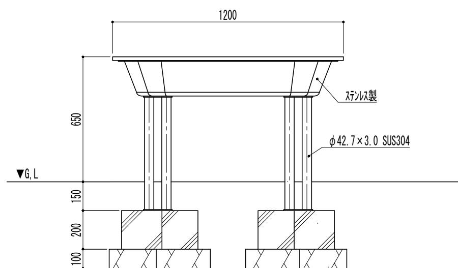
正面図
