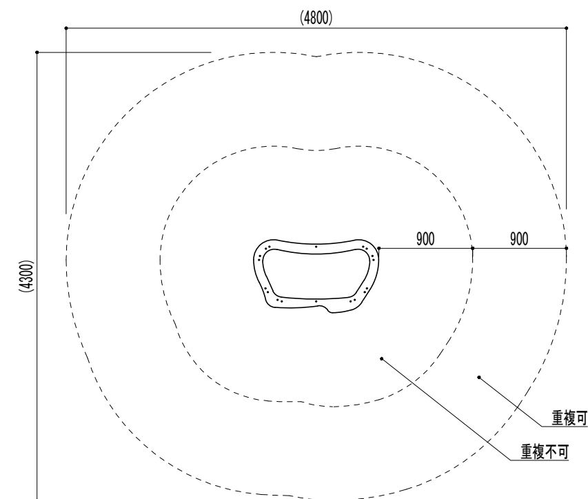
安全領域図 S=1/50
