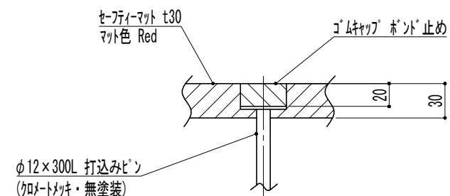
セーフティーマット詳細図
