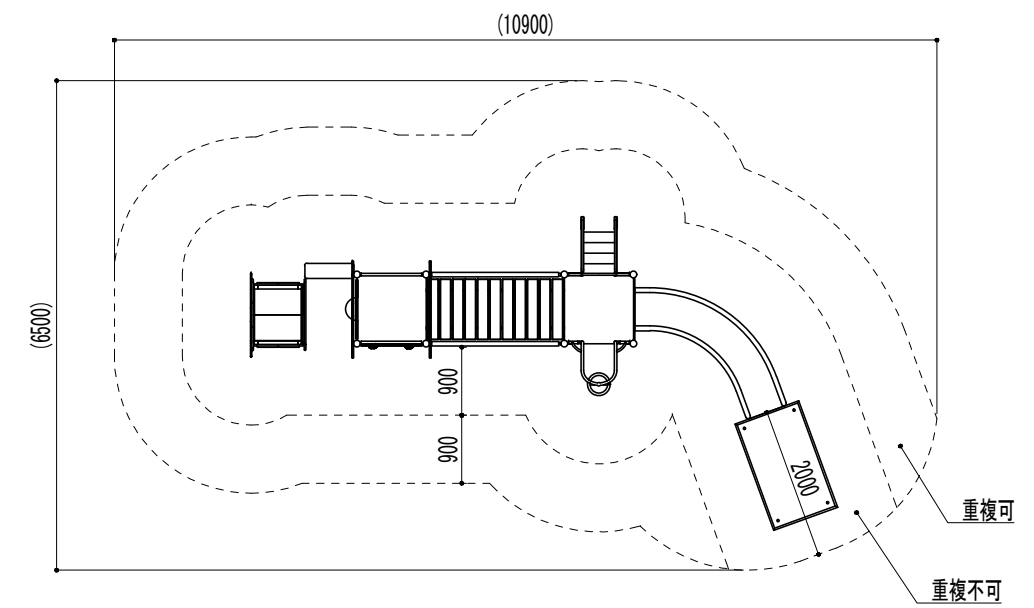
安全領域図 S=1/100
