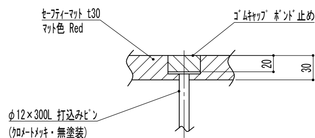
セーフティーマット詳細図
