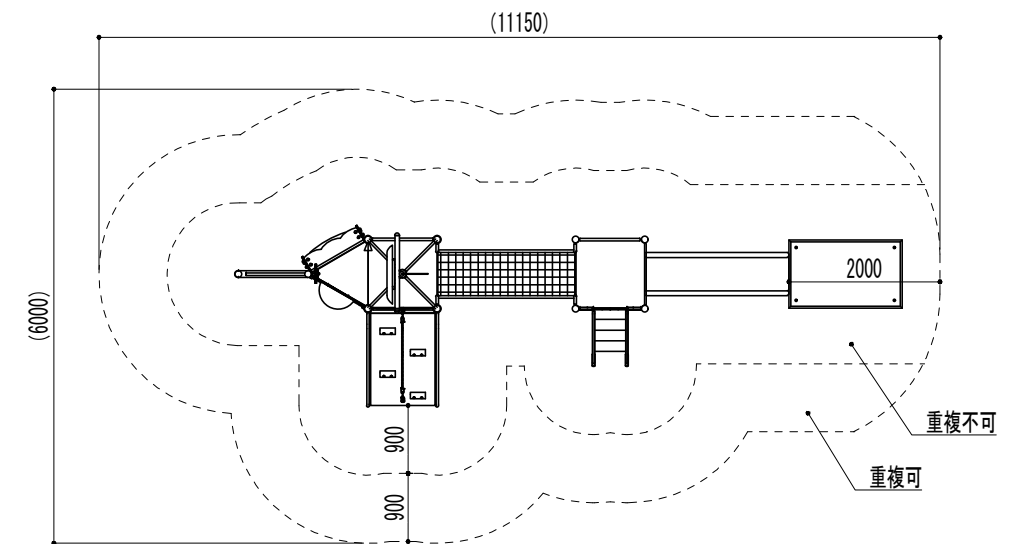
安全領域図 S=1/100
