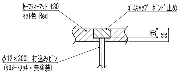
セーフティーマット詳細図
