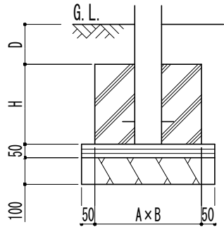
基礎詳細図
