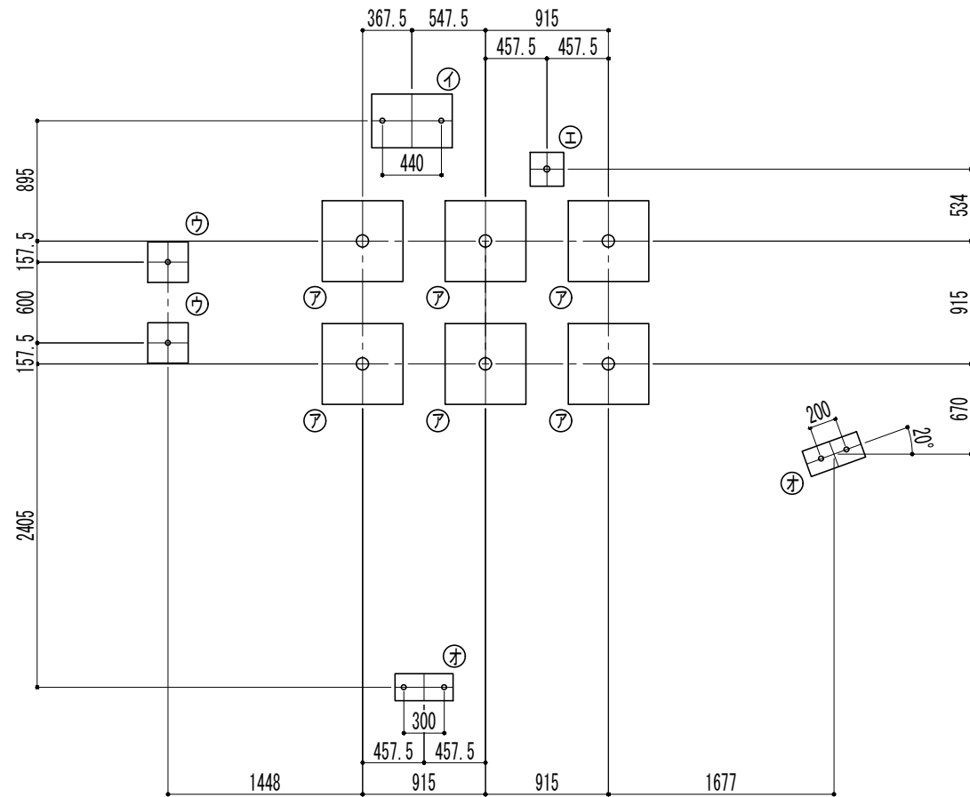
基礎伏図
