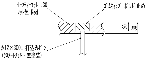
セーフティマット詳細図
