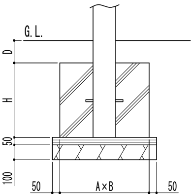
基礎詳細図
