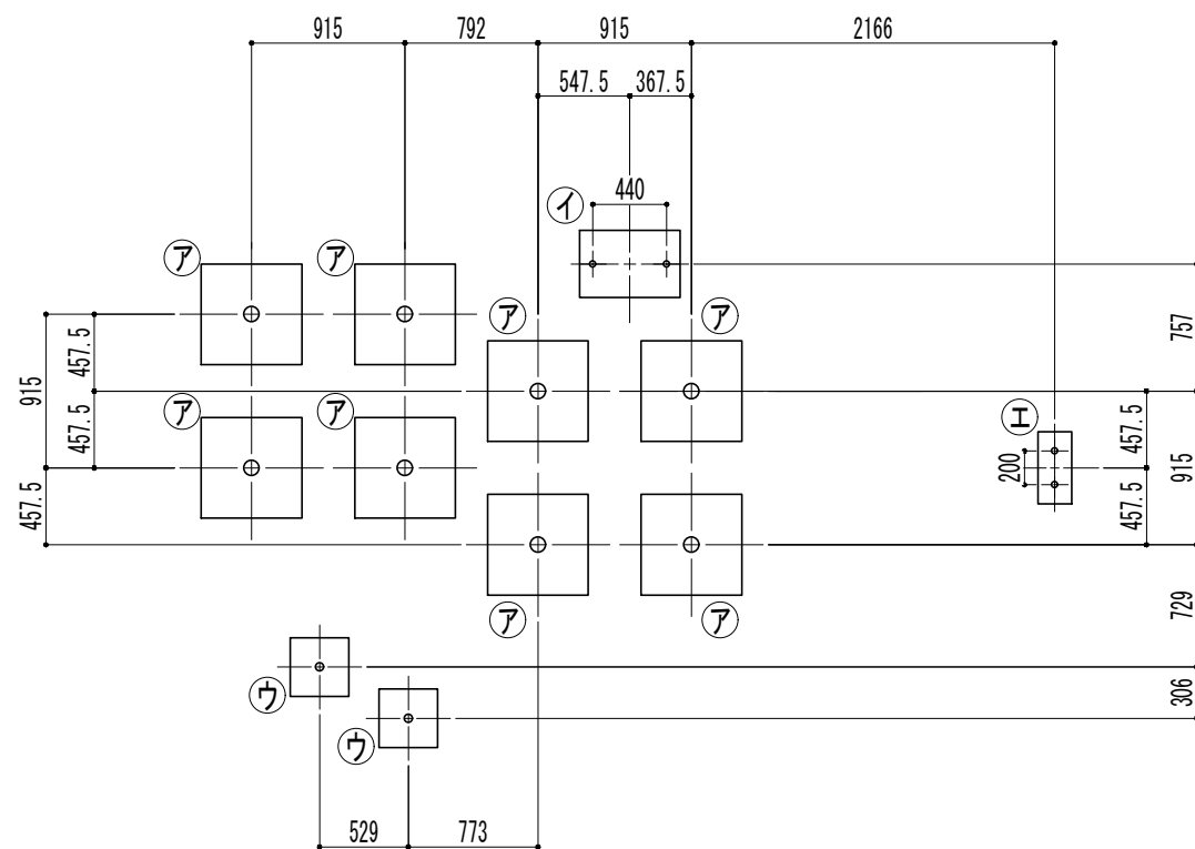
基礎伏図
