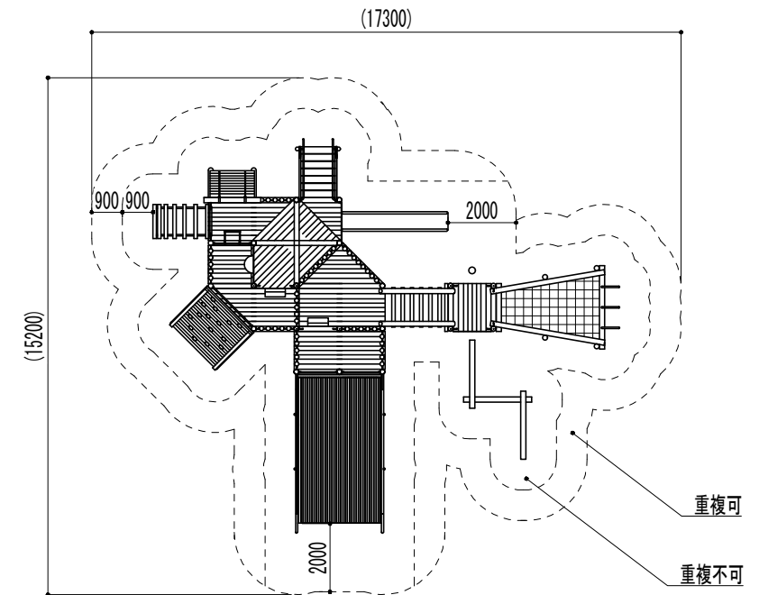
安全領域図 S=1/200
