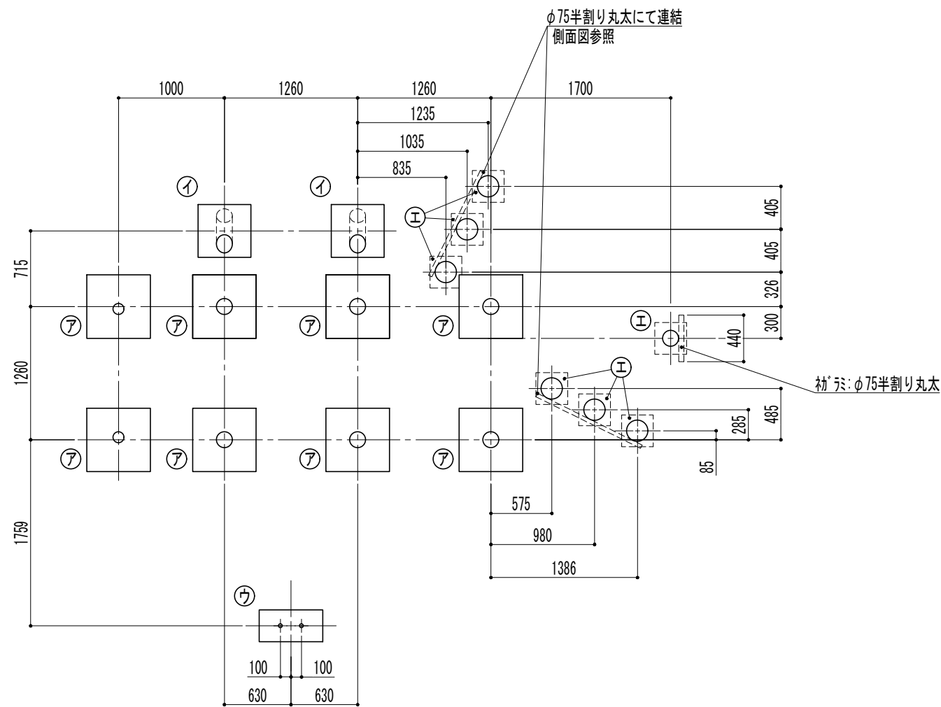
基礎伏図
