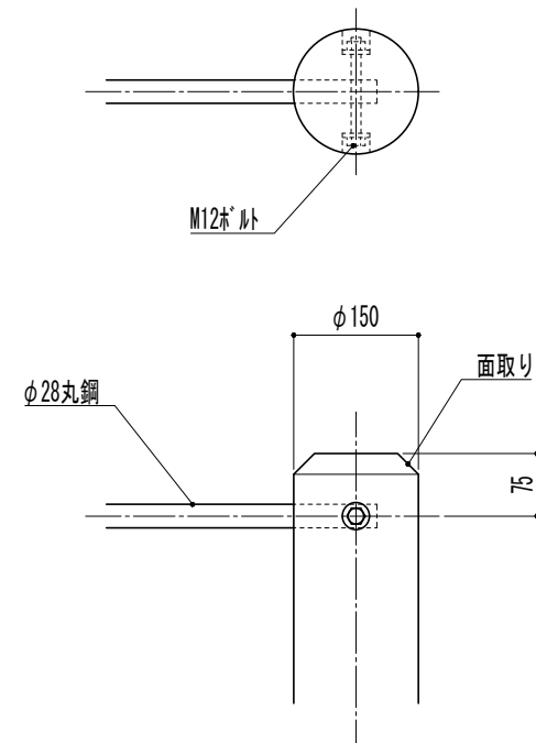
鉄棒取付け詳細図 S=1/10
