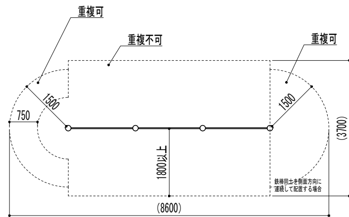
安全領域図 S=1/100
